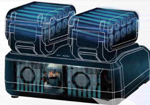
Built-in fan
